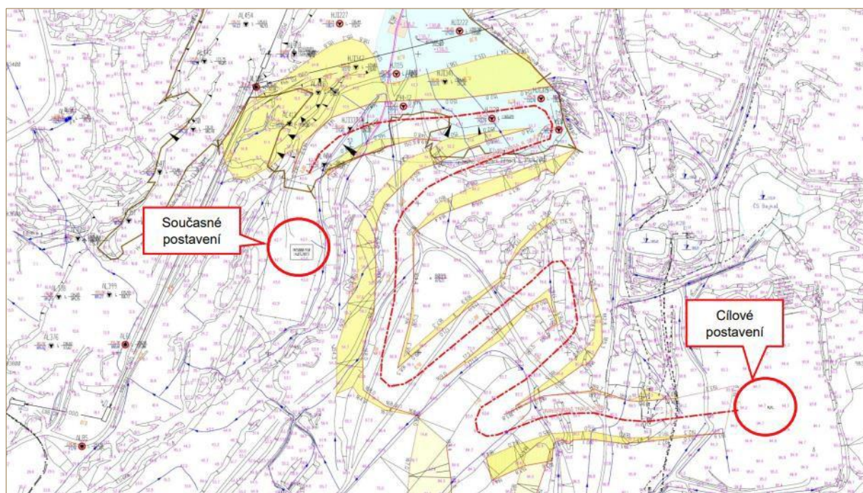
Obrázek 20: Transportní trasa rypadla.
