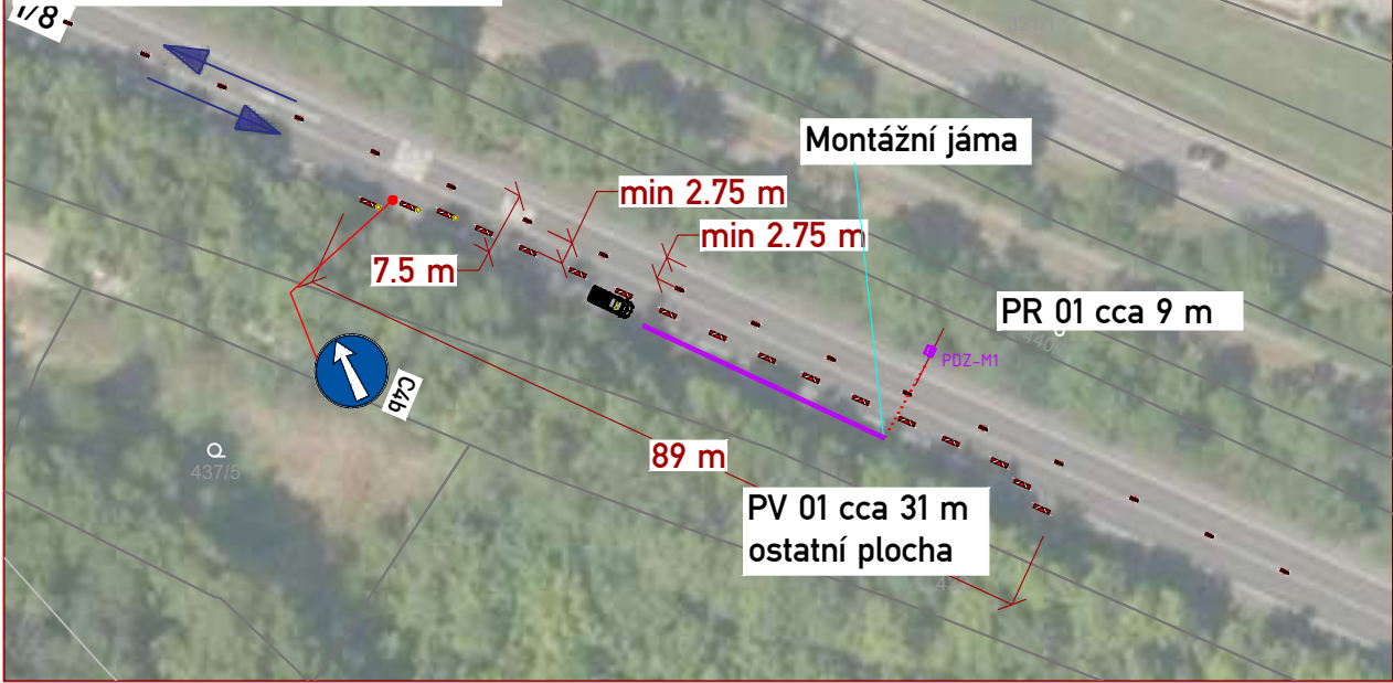
Detail - pracovní místo (1:1000)
